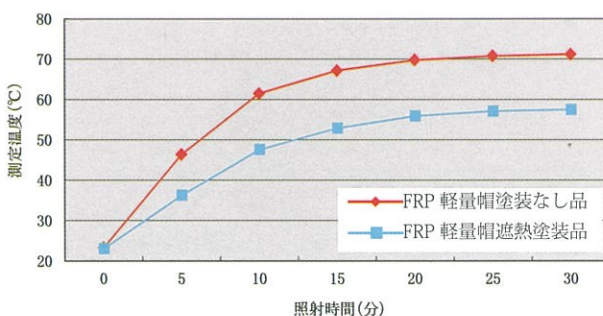
【遮熱塗装有・無による温度比較 (FRP 軽量)】
